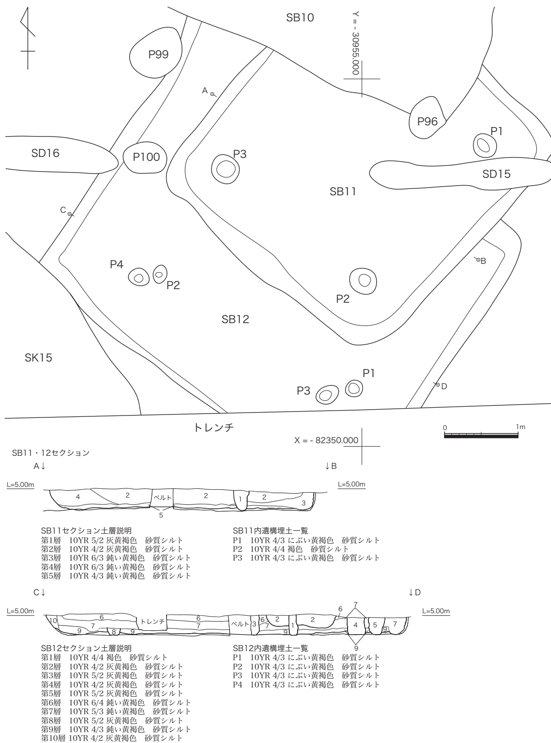
第 17 図 竪穴建物跡 S B 11・12 遺構図 (S=1:50)
