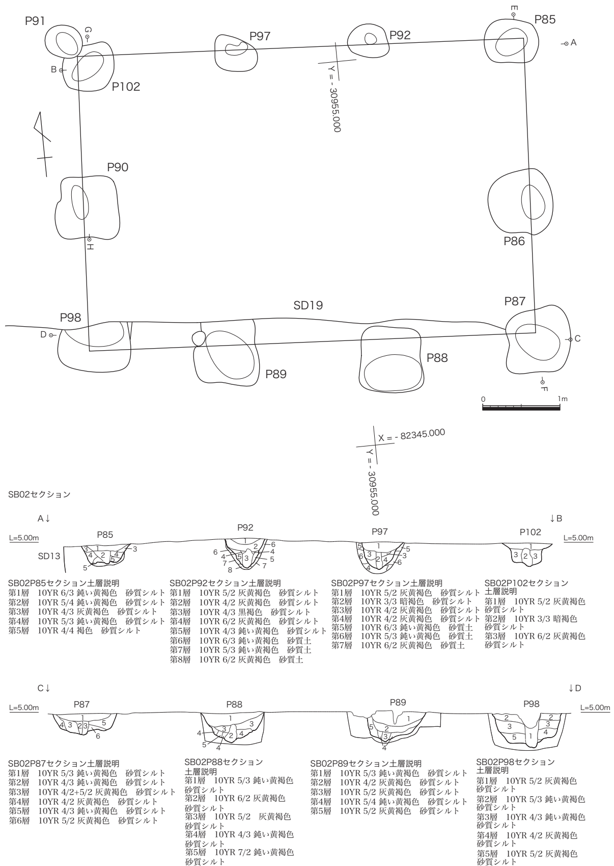
第 68 図 掘立柱建物跡 S B 02 遺構図 (1) (S=1:50)
