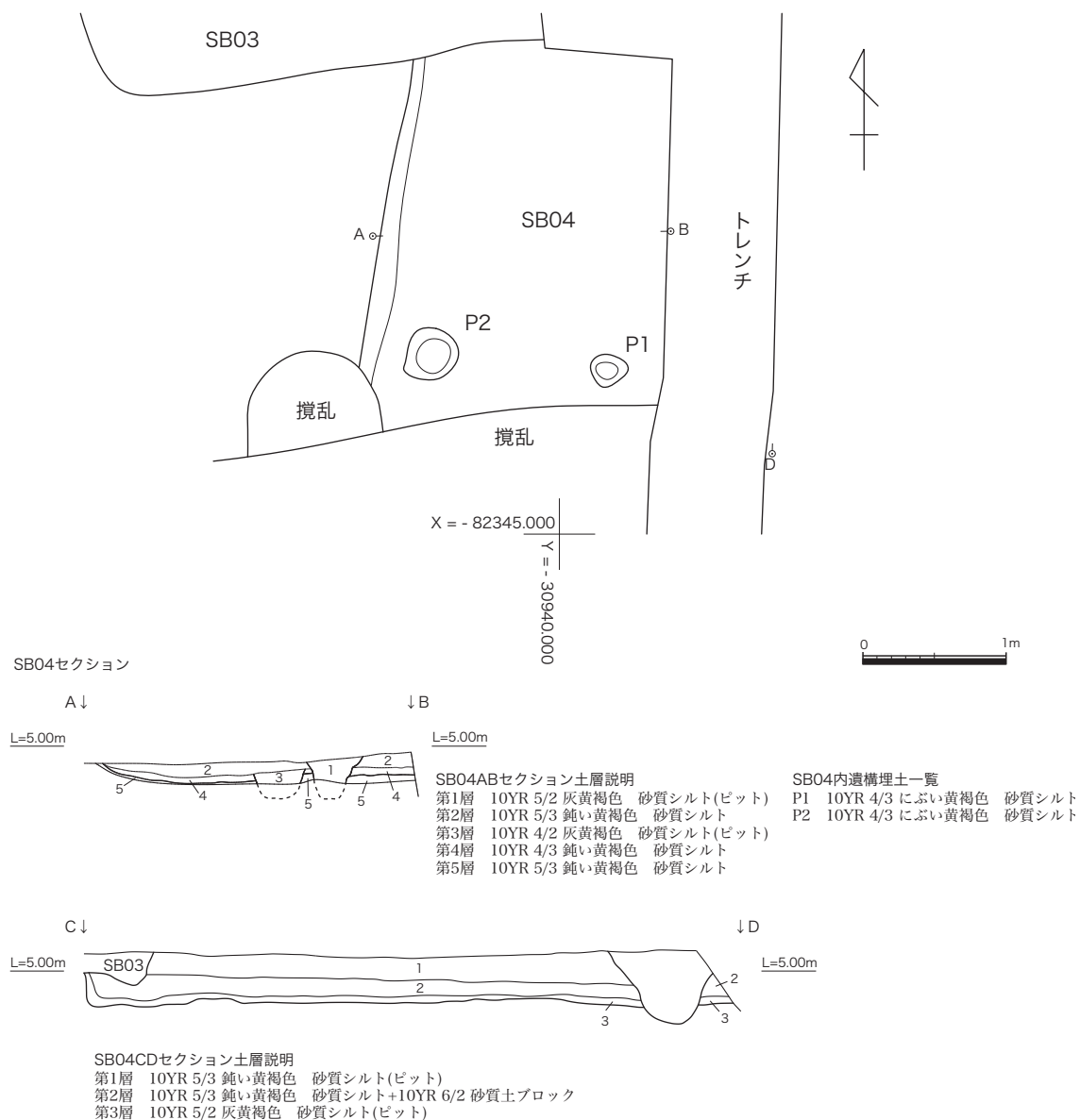
第 11 図 竪穴建物跡 S B 04 遺構図 (S=1:50)
