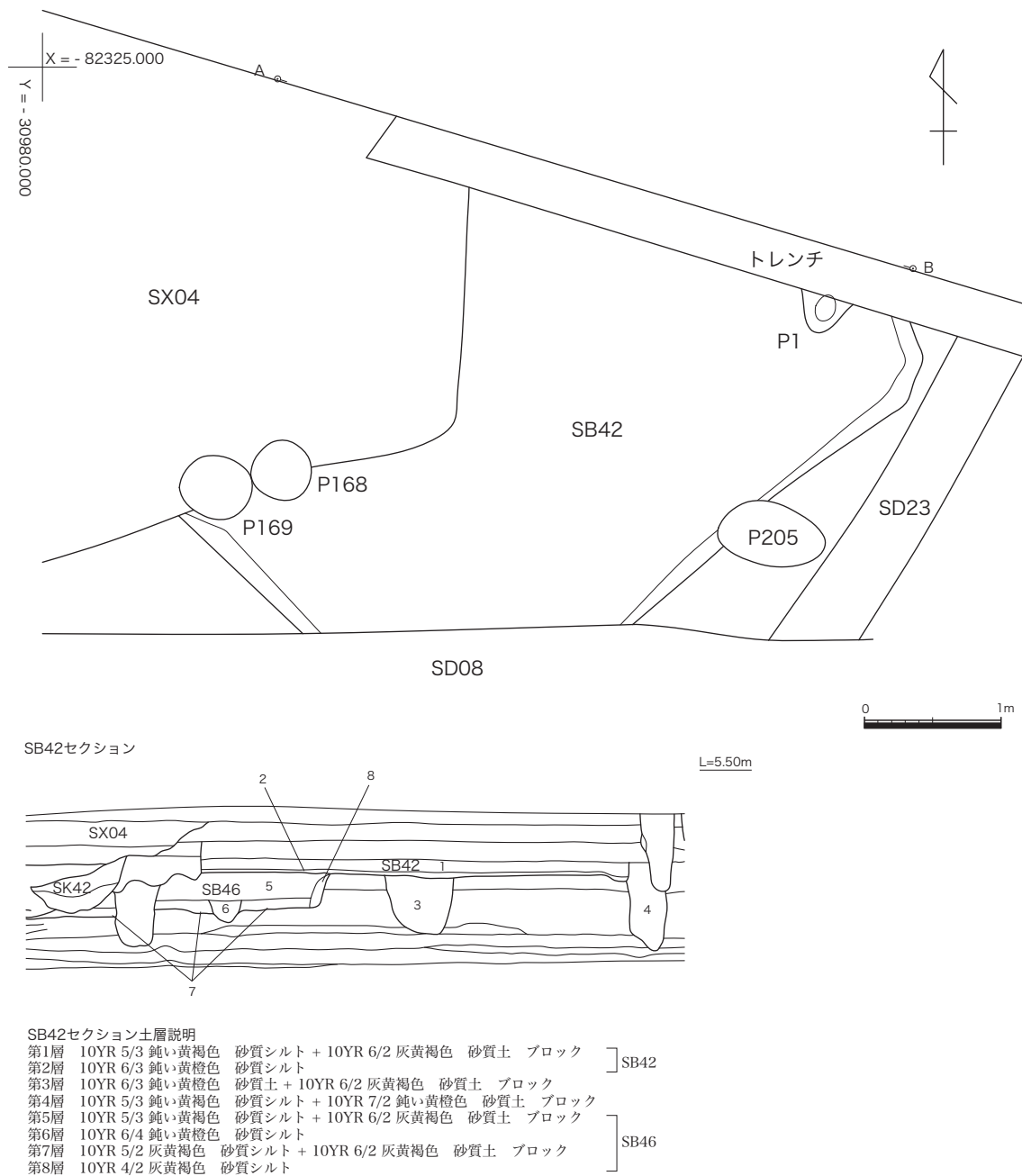
第 43 図 竪穴建物跡 S B 42 遺構図 (S=1:50)
