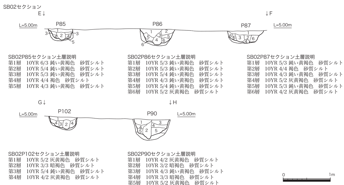
第 69 図 掘立柱建物跡 S B 02 遺構図 (2) (S=1:50)
