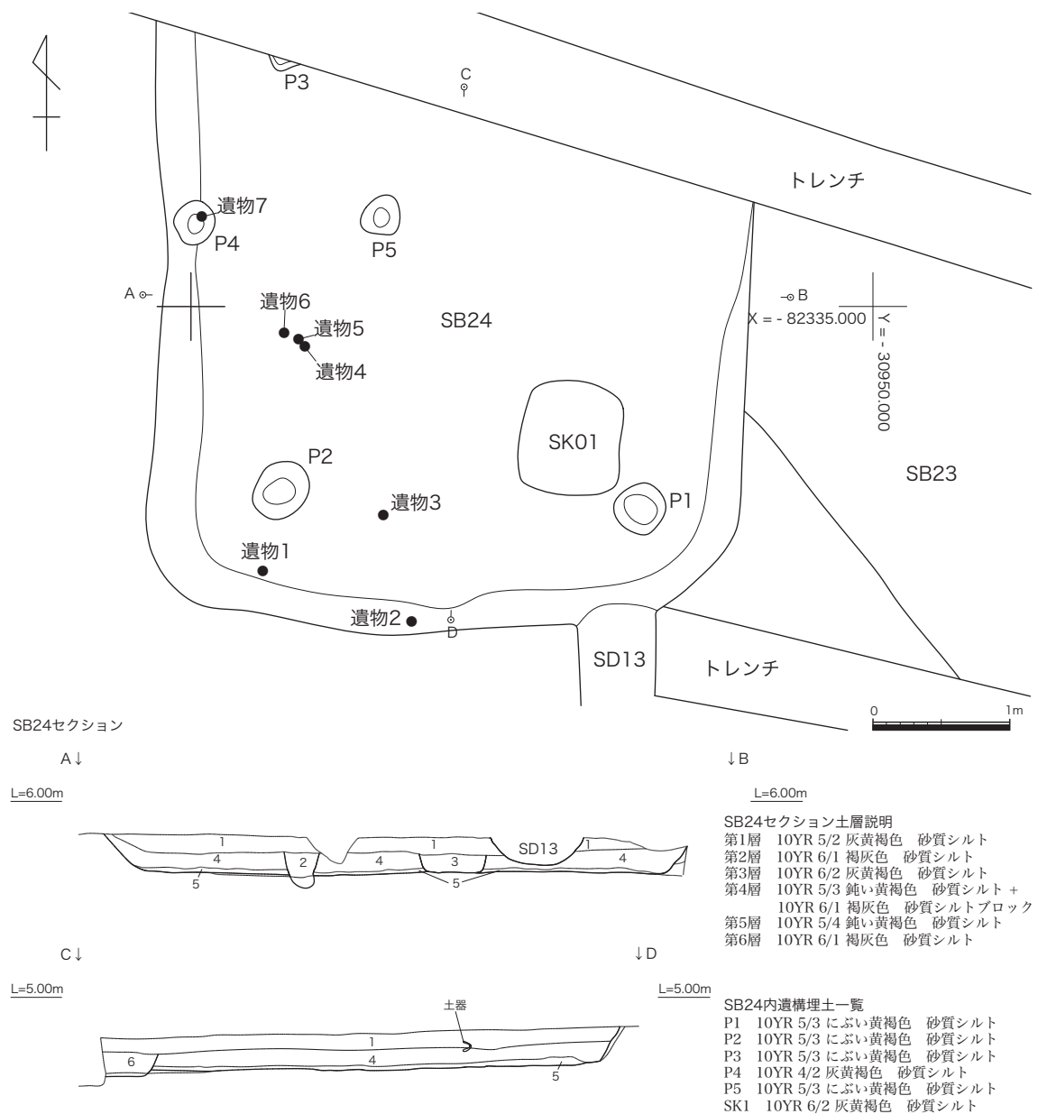
第 28 図 竪穴建物跡 S B 24 遺構図 (S=1:50)
