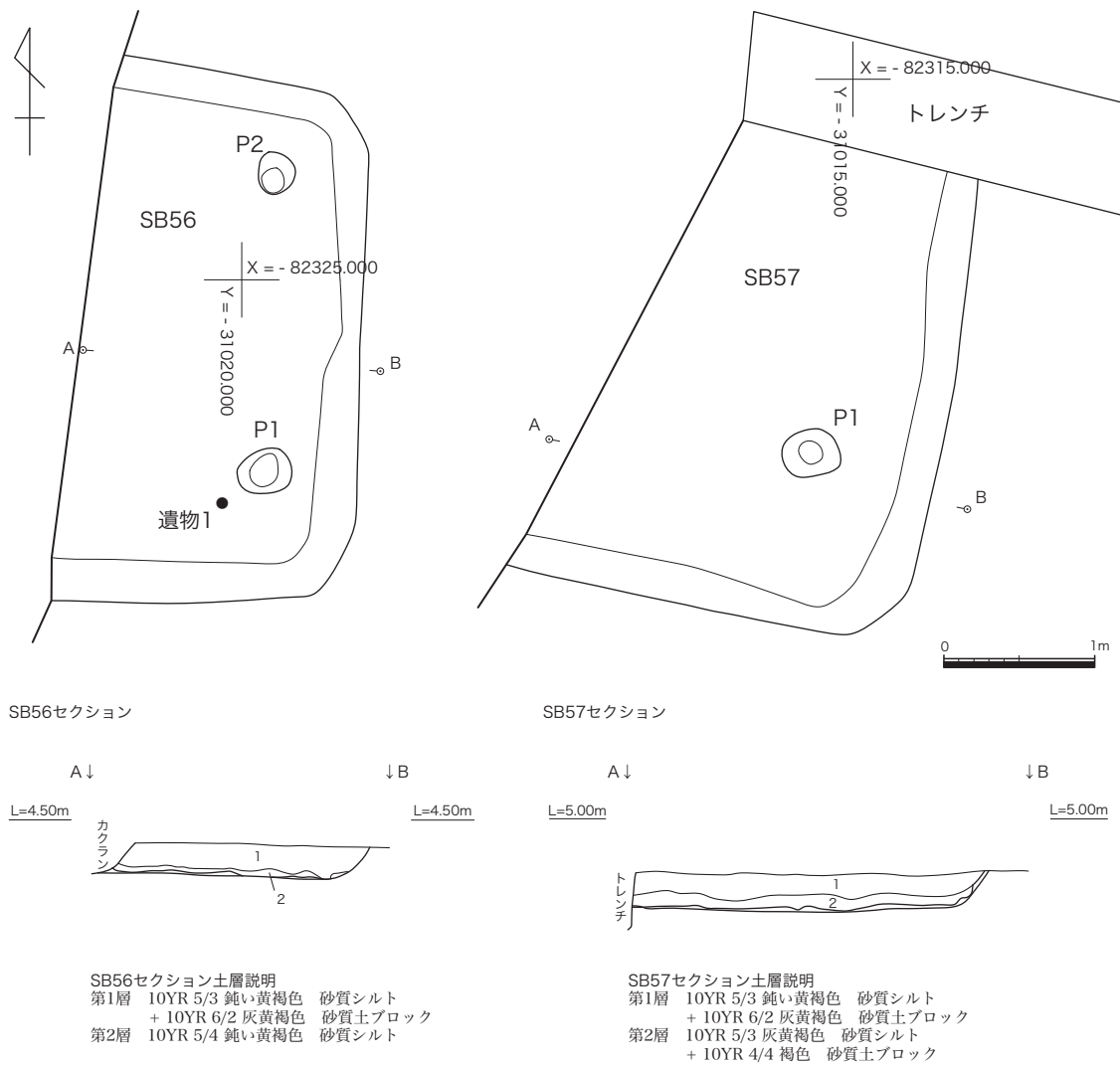
第 51 図 竪穴建物跡 S B 56・57 遺構図 (S=1:50)
