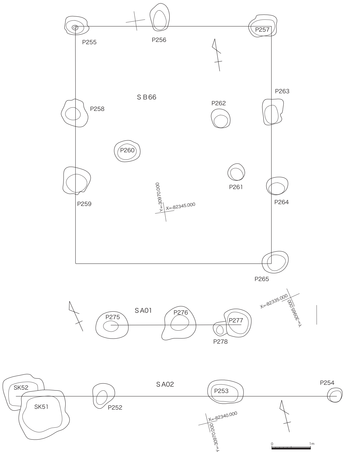
第 63 図 掘立柱建物跡 S B 66、SA01・02 遺構図 (S=1:50)
