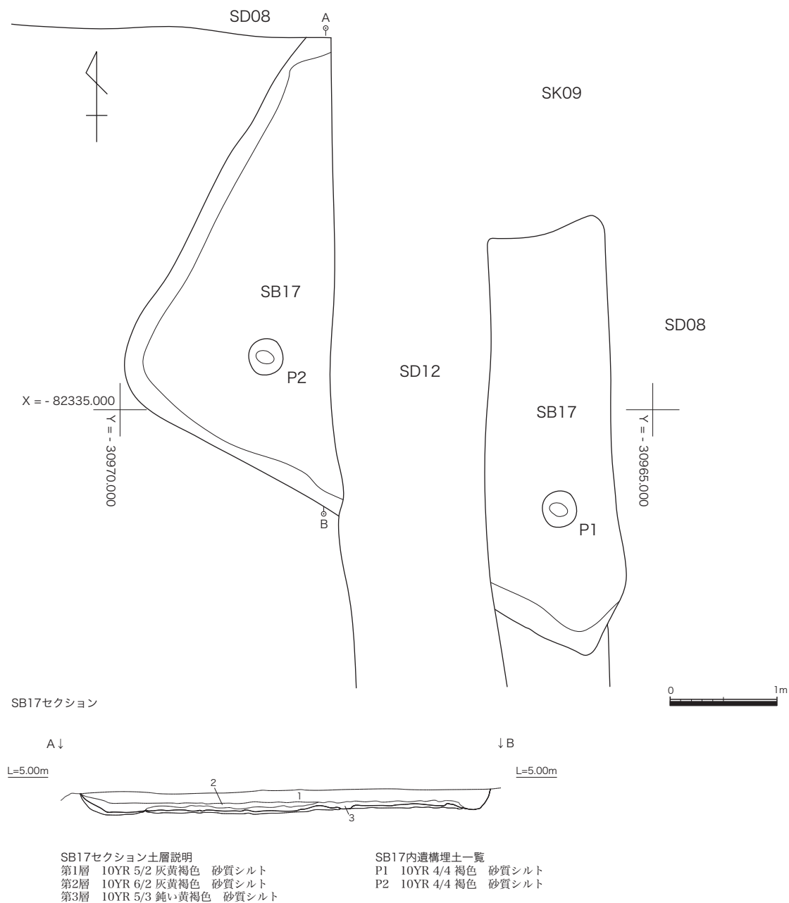
第 21 図 竪穴建物跡 S B 17 遺構図 (S=1:50)
