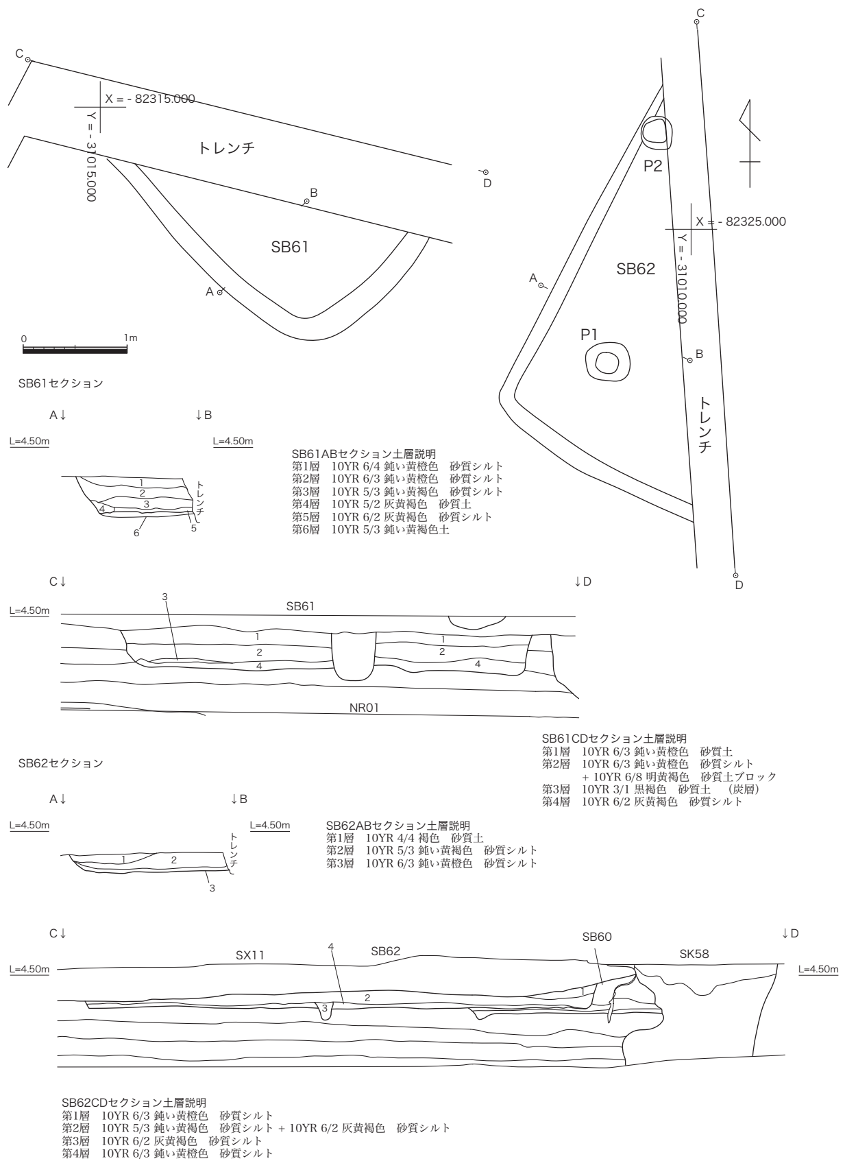
第 55 図 竪穴建物跡 S B 61・62 遺構図 (S=1:50)
