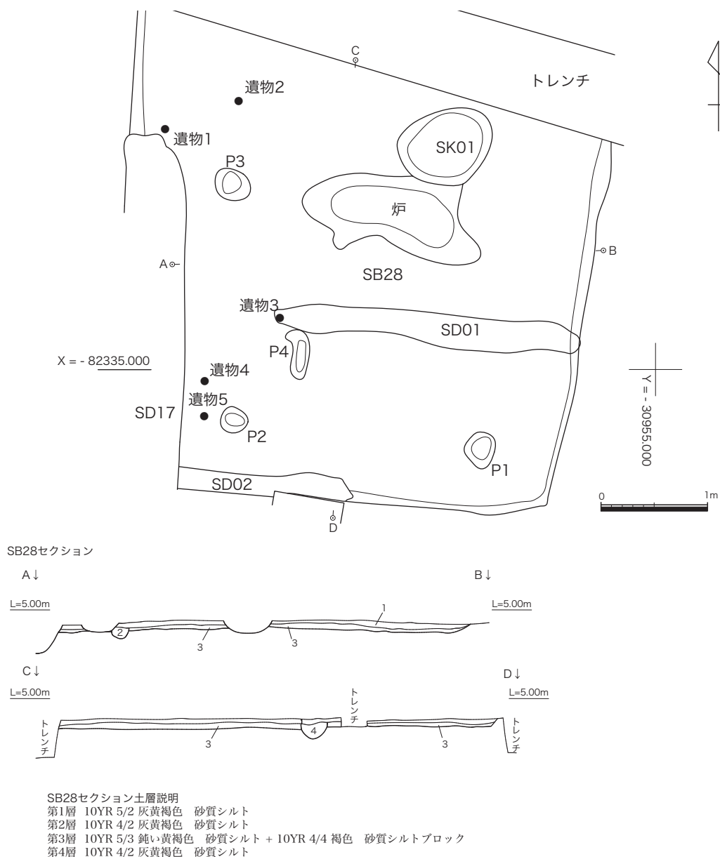
第 32 図 竪穴建物跡 S B 28 遺構図 (S=1:50)
