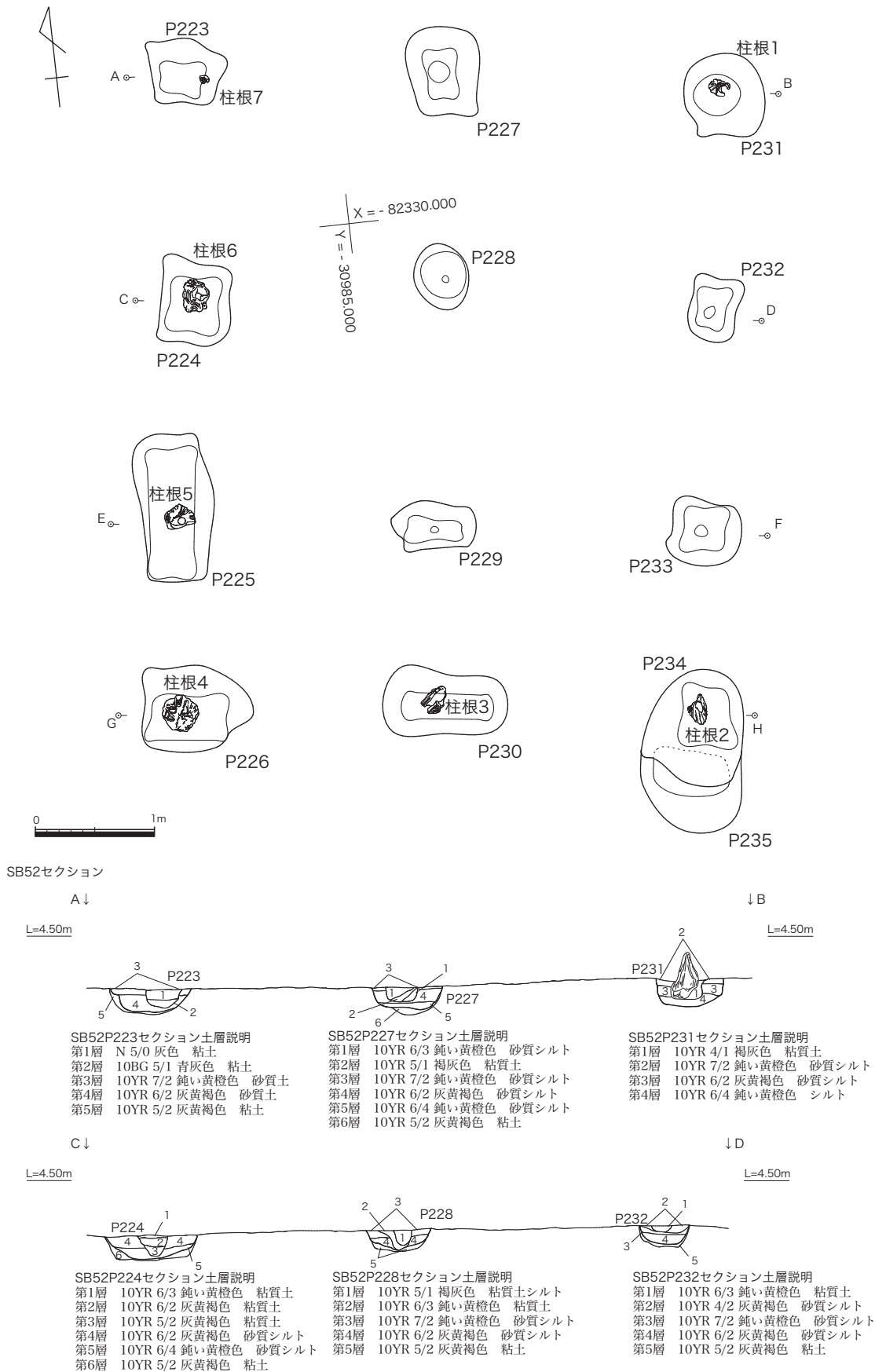
第 59 図 掘立柱建物跡 S B 52 遺構図 (1) (S=1:50)
