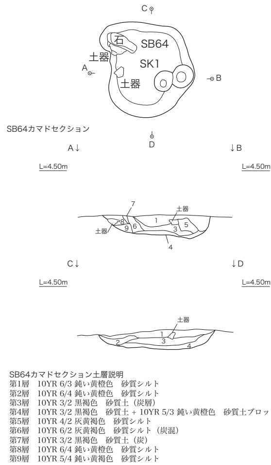
第 58 図 竪穴建物跡 S B 64・65 遺構図 (2)
