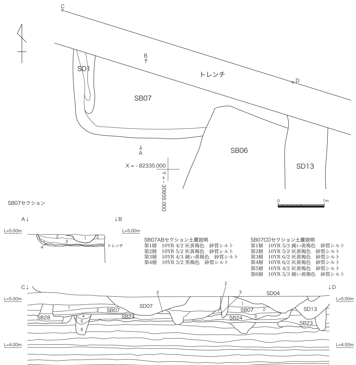
第 14 図 竪穴建物跡 SB 07 遺構図 (S=1:50)
