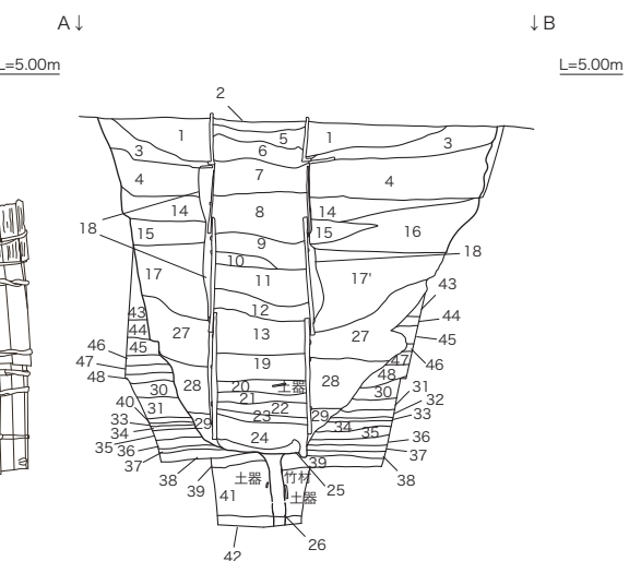
第 76 図 井戸 S K 58・65 遺構図 (S=1:50)
