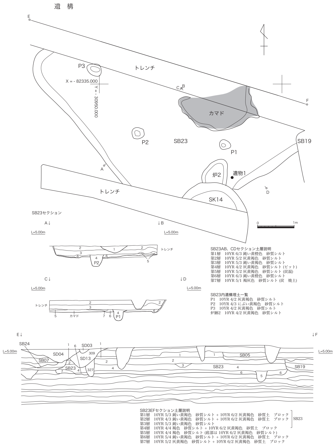
第26図 竪穴建物跡S B 23 遺構図 (S=1:50)
