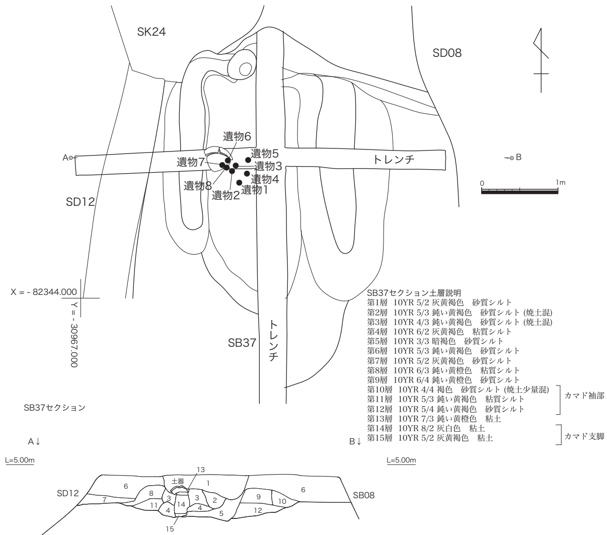
第 35 図 竪穴建物跡 S B 37 遺構図 (S=1:50)
