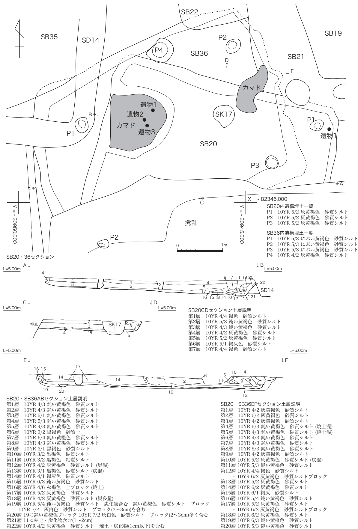
第 25 図 竪穴建物跡 S B 20・36 遺構図 (S=1:50)
