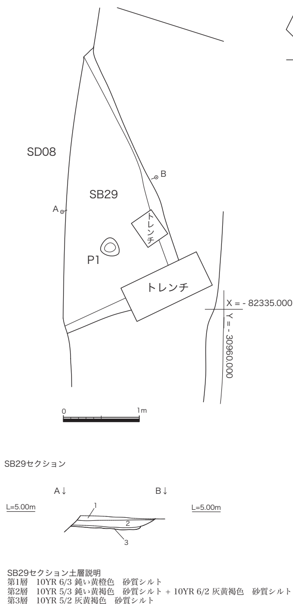
第 33 図 竪穴建物跡 S B 29 遺構図 (S=1:50)
