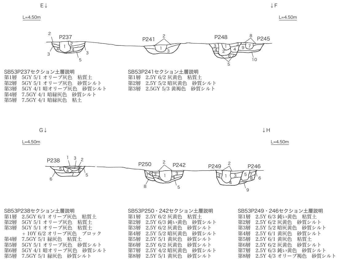
第 62 図 掘立柱建物跡 S B 53 遺構図（2）（S=1:50）
