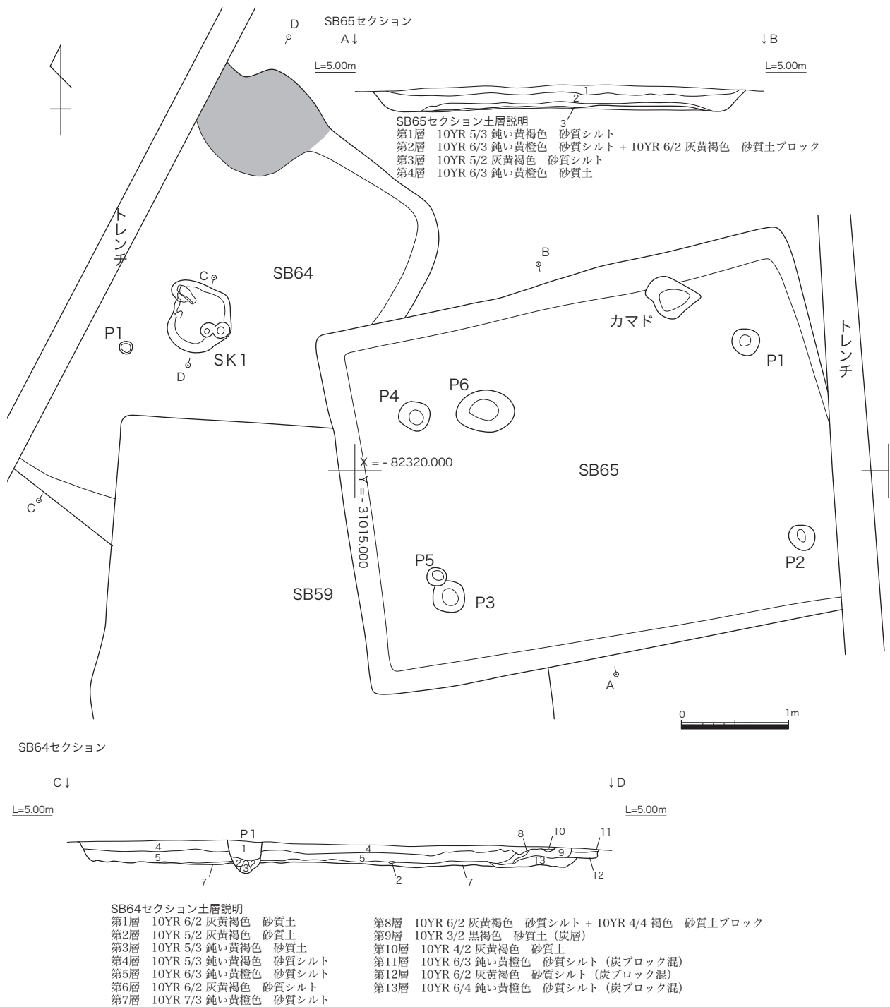
第 57 図 竪穴建物跡 S B 64・65 遺構図 (1) (S=1:50)
