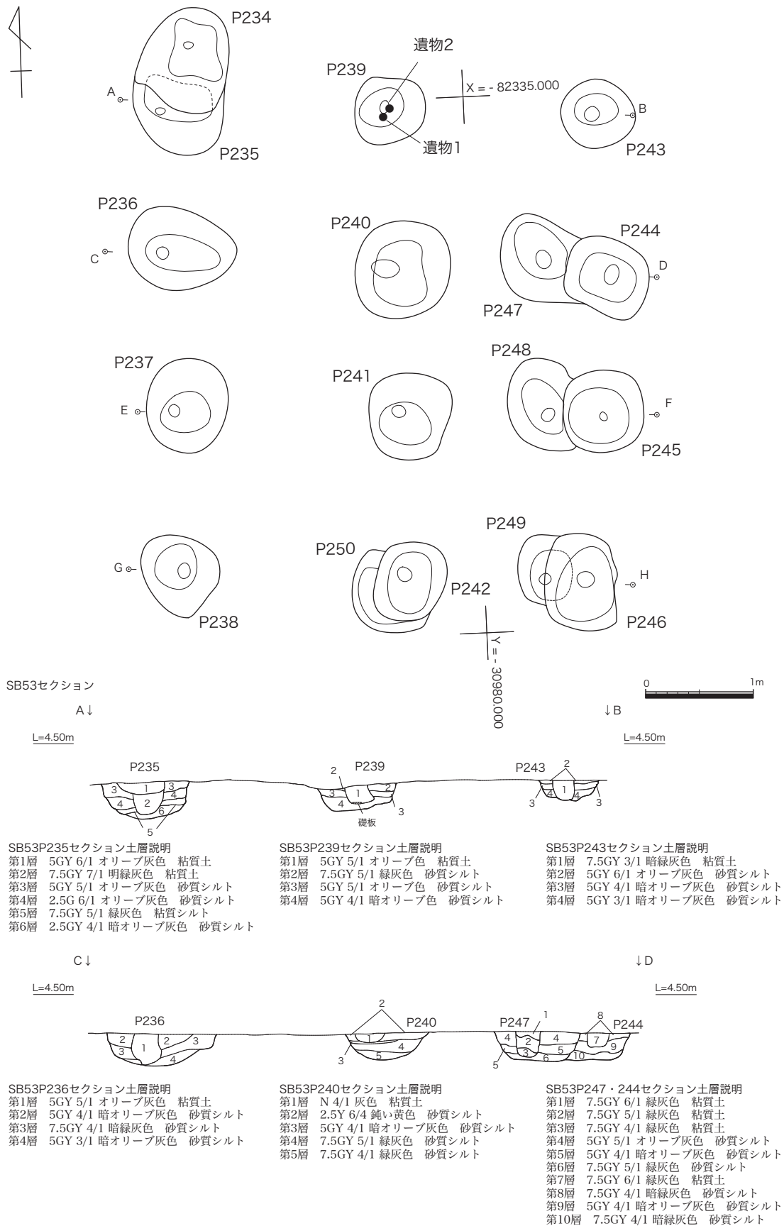
第 61 図 掘立柱建物跡 S B 53 遺構図 (1) (S=1:50)
