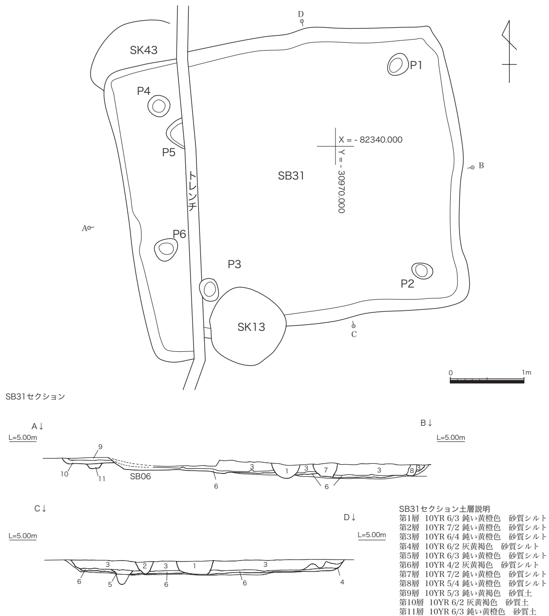
第 36 図 竪穴建物跡 S B 31 遺構図 (S=1:50)
