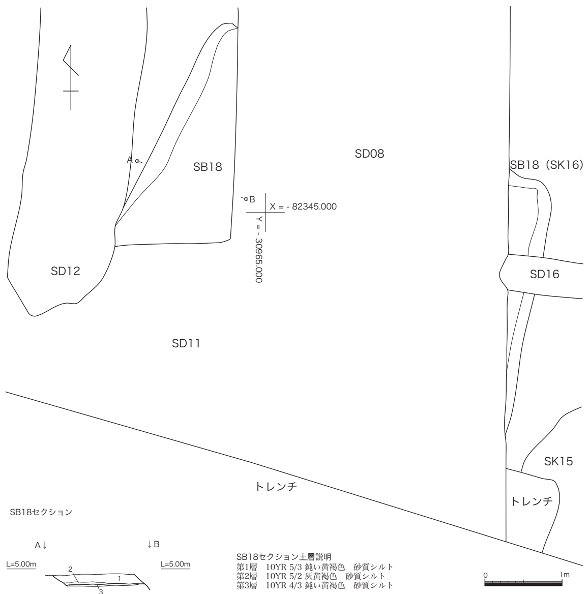
第22図 竪穴建物跡S B 18 遺構図 (S=1:50)
