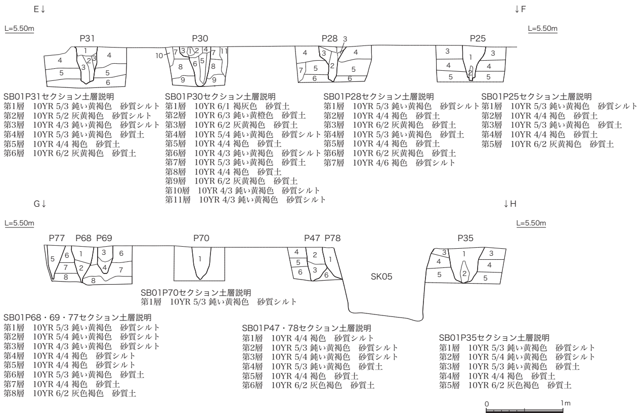
第 67 図 掘立柱建物跡 S B 01 遺構図（2）（S=1:50）
