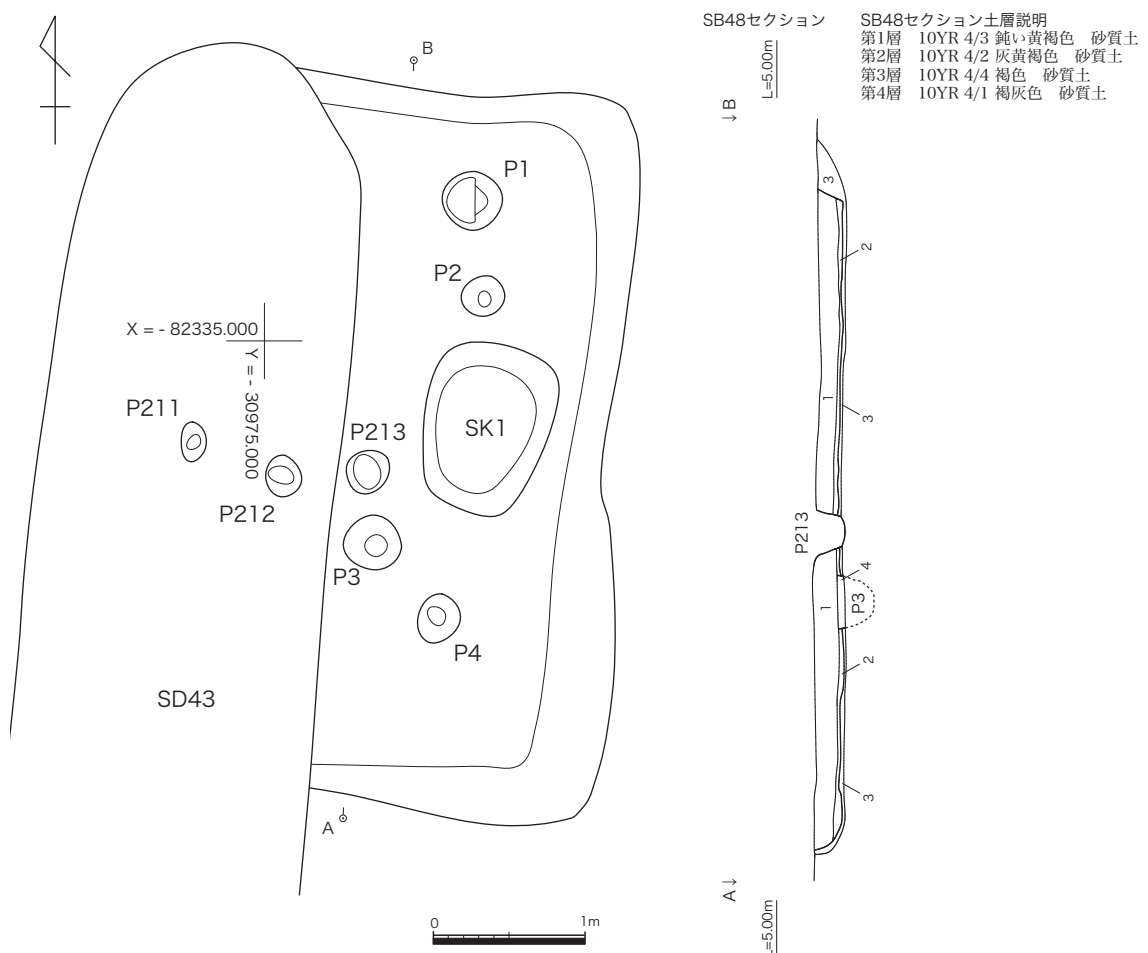
第 46 図 竪穴建物跡 S B 48 遺構図 (S=1:50)
