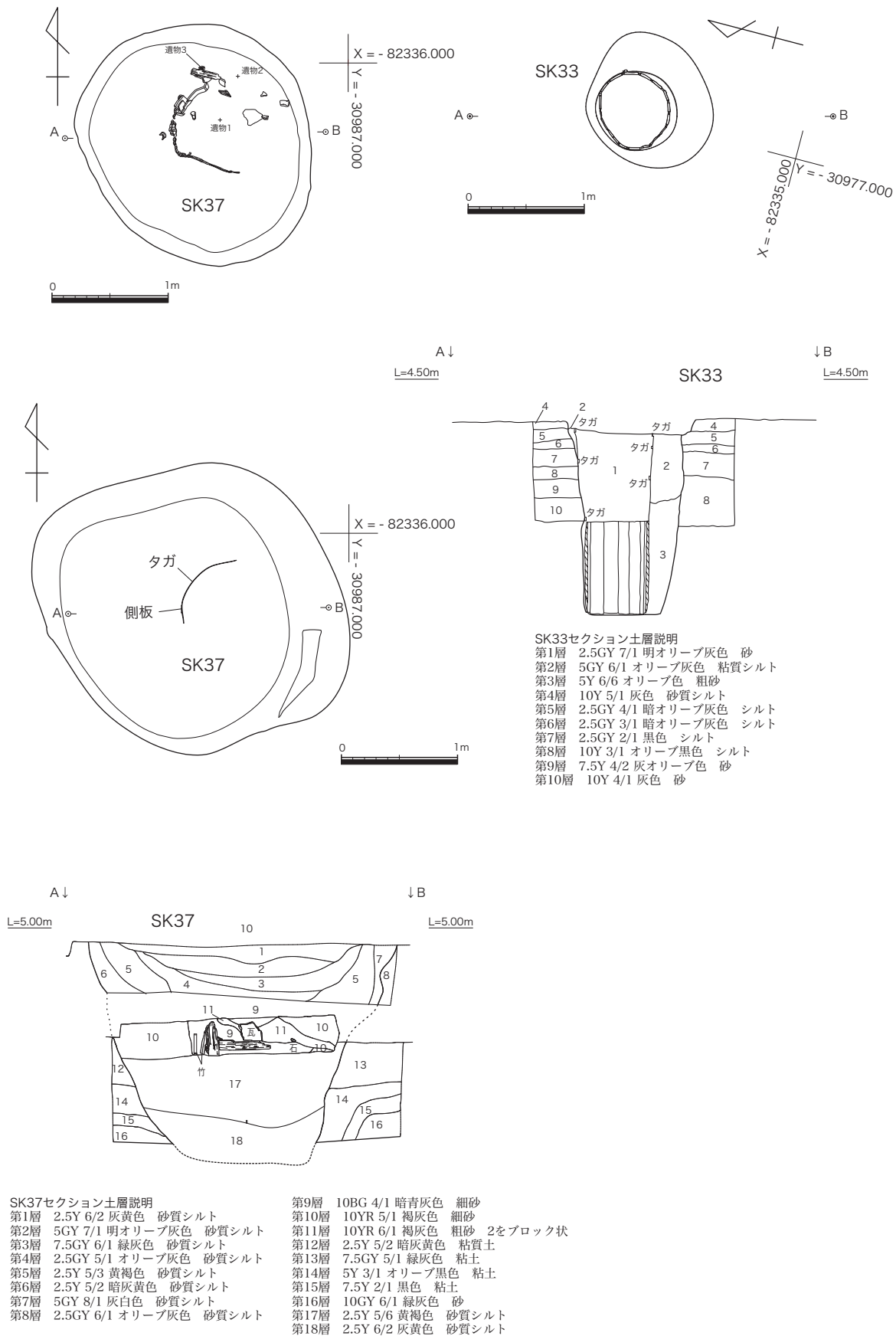
第 75 図 井戸 S K 33・37 遺構図 (S=1:50)
