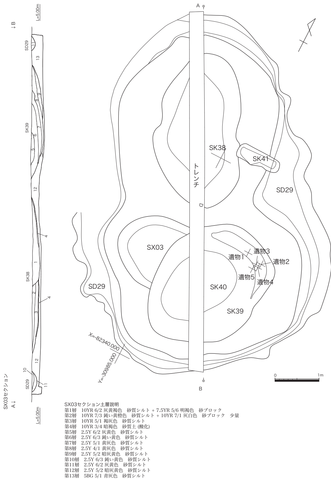
第 77 図 S X 03 遺構図 (S=1:50)
