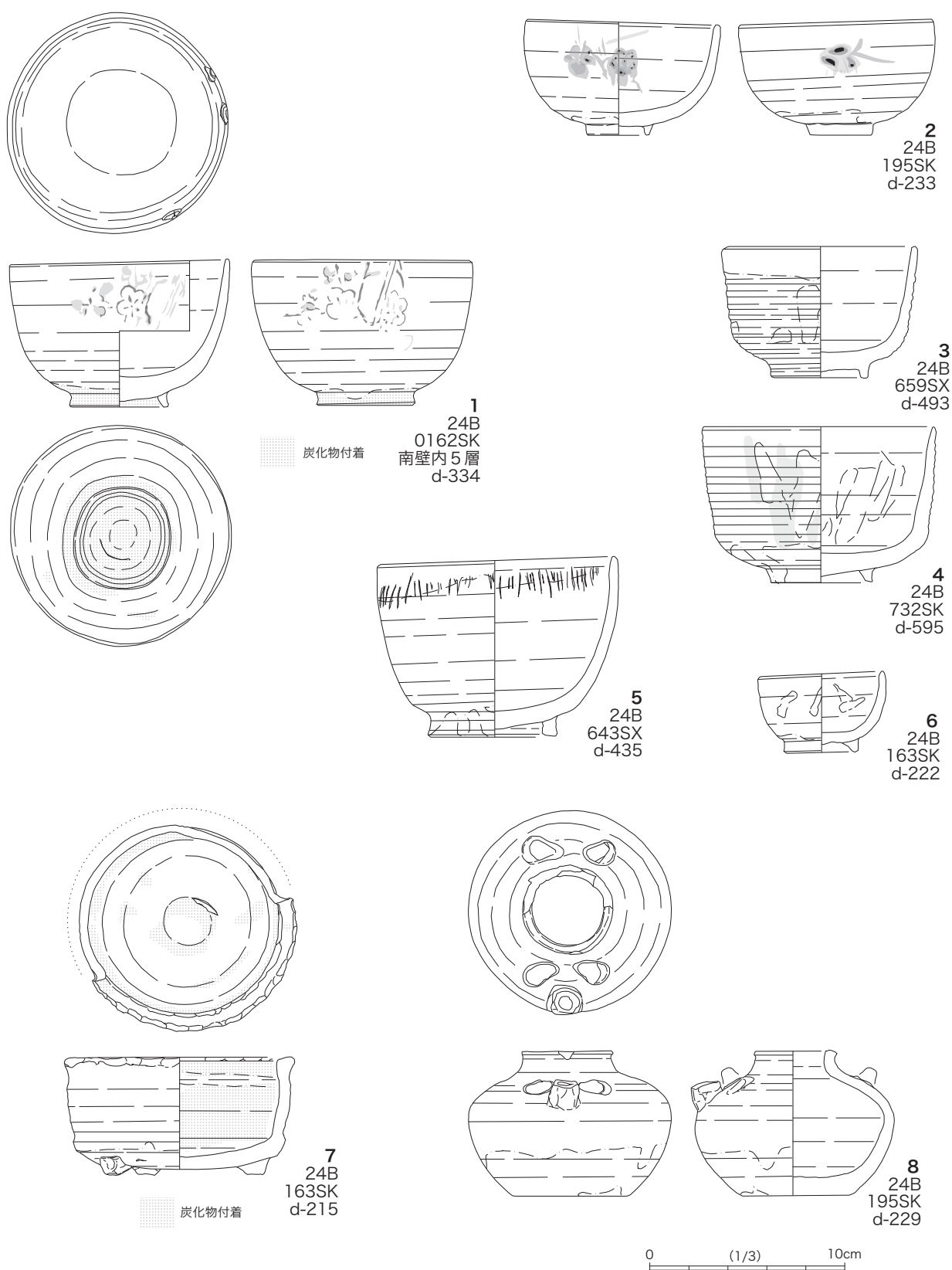
図8 西二葉町遺跡出土 近世遺物1【24B区】
