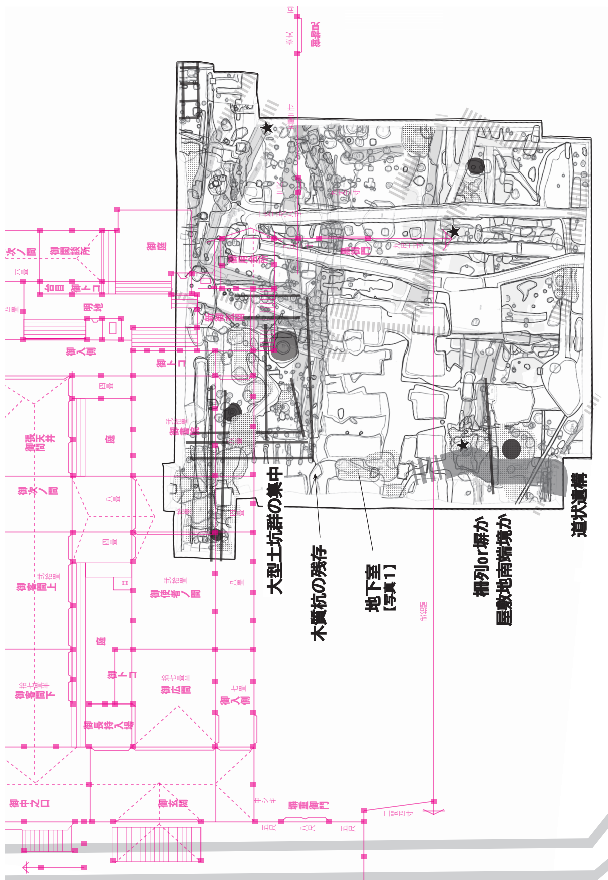
図7 成瀬隼人正中屋敷絵図と道跡調査平面図との関係4 (1/300)
