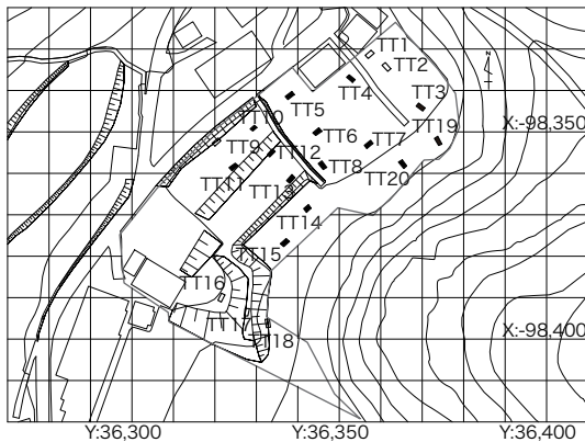
■ 遺構・遺物が確認された試掘坑 テストトレンチ配置 (1:2000)
