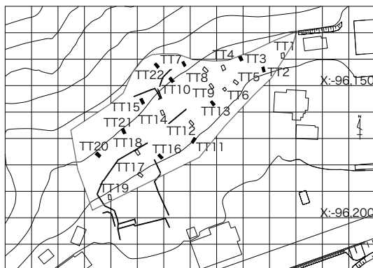
遺構・遺物が確認された試掘坑 テストトレンチ配置 (1:2000)
