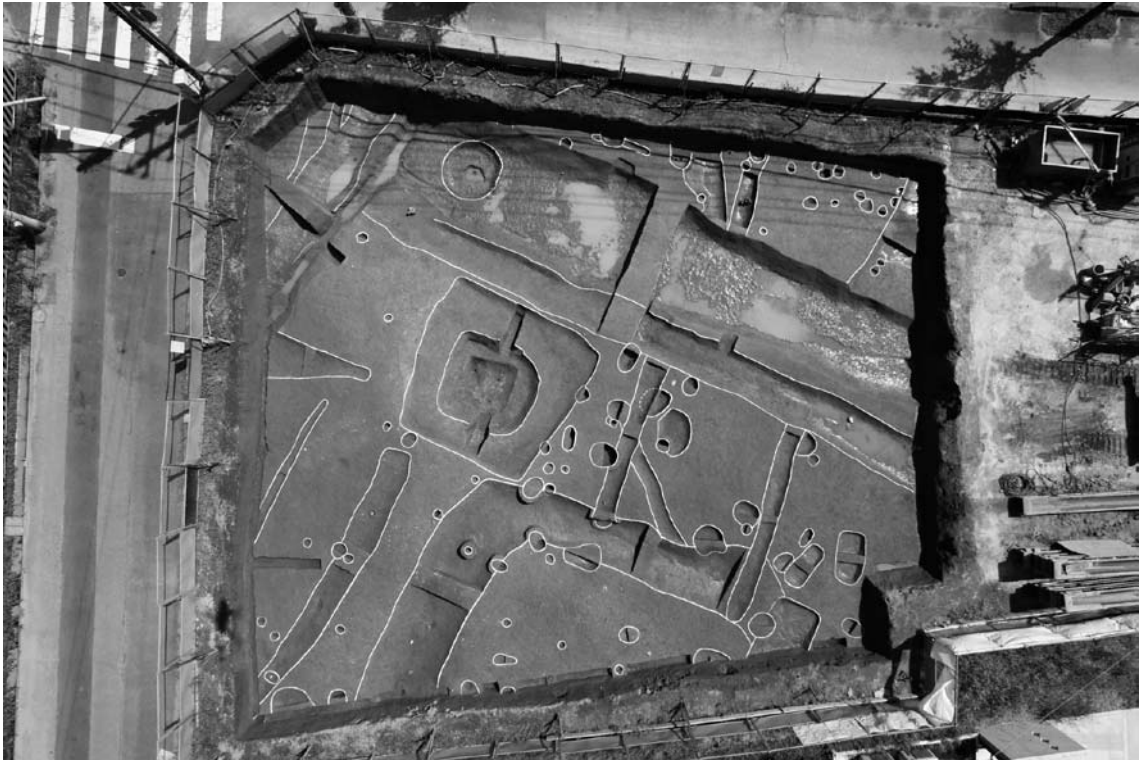
09C 区全景（上空から）
