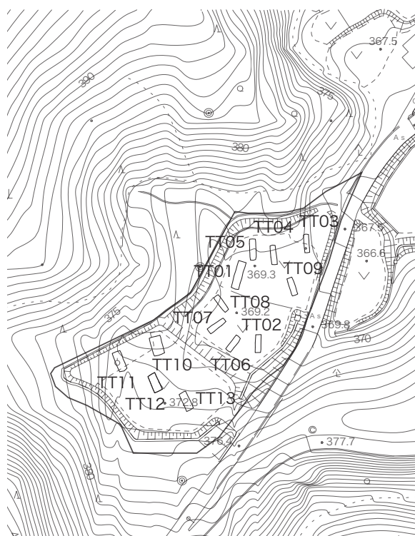
神谷上切遺跡トレンチ配置図(1:1500)
