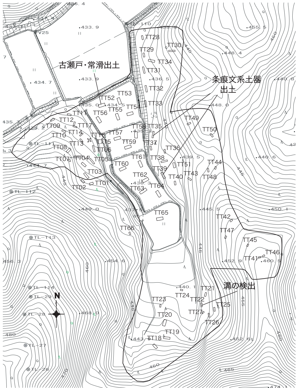
朴の木トレンチ配置図 (1:1500)
