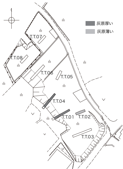
八巻古窯群テストトレンチ配置図 (1/500)
