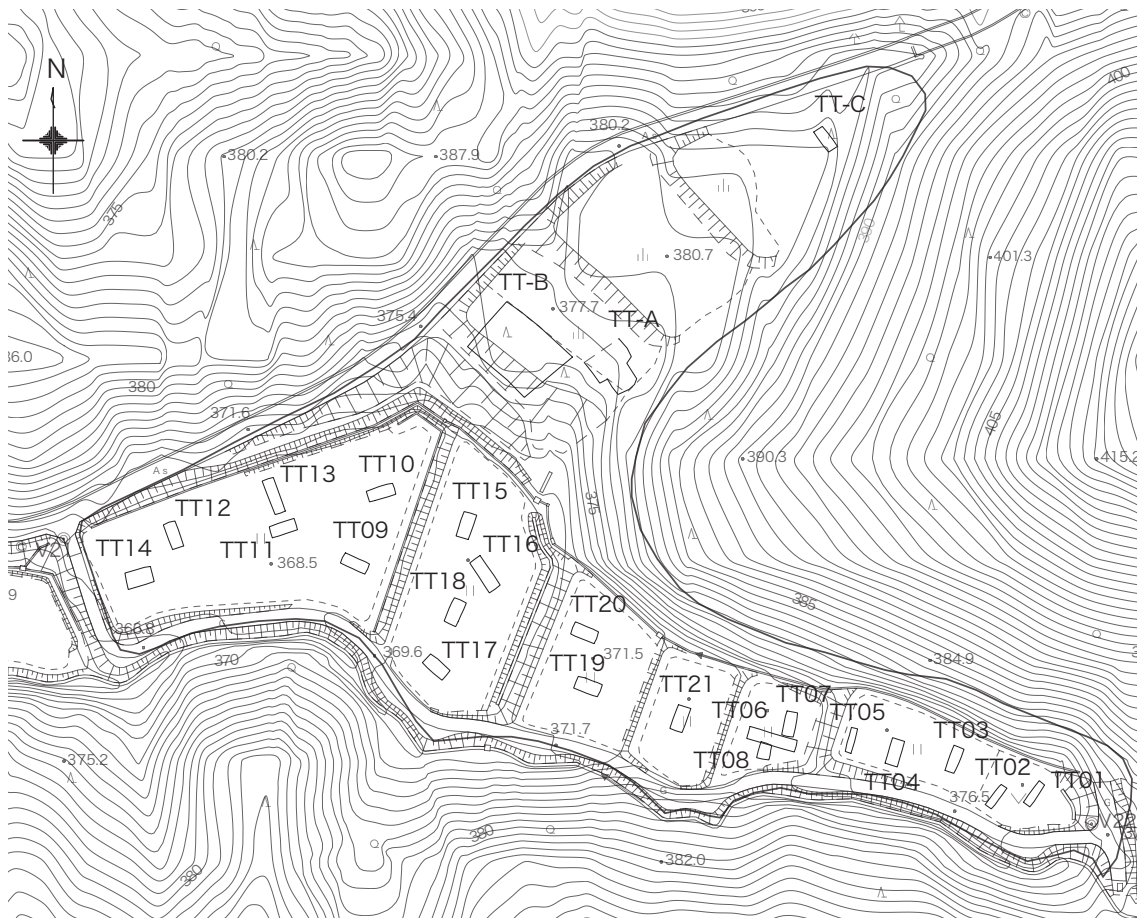
中坂佐後遺跡トレンチ配置図(1:1500)
