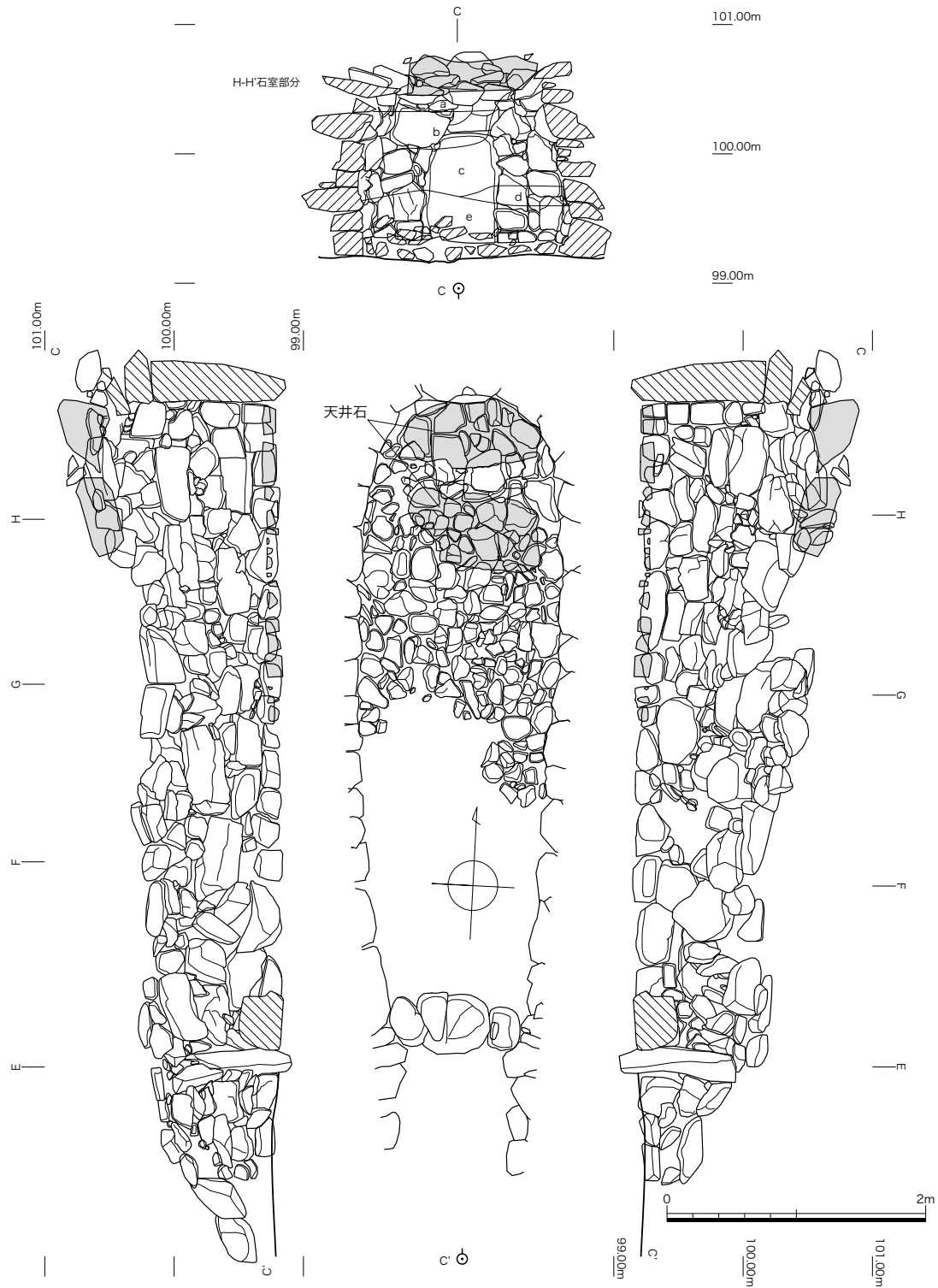
石室平面・立面展開図 (1:50)
