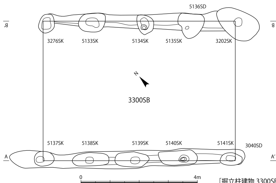
〔掘立柱建物 3300SB〕
