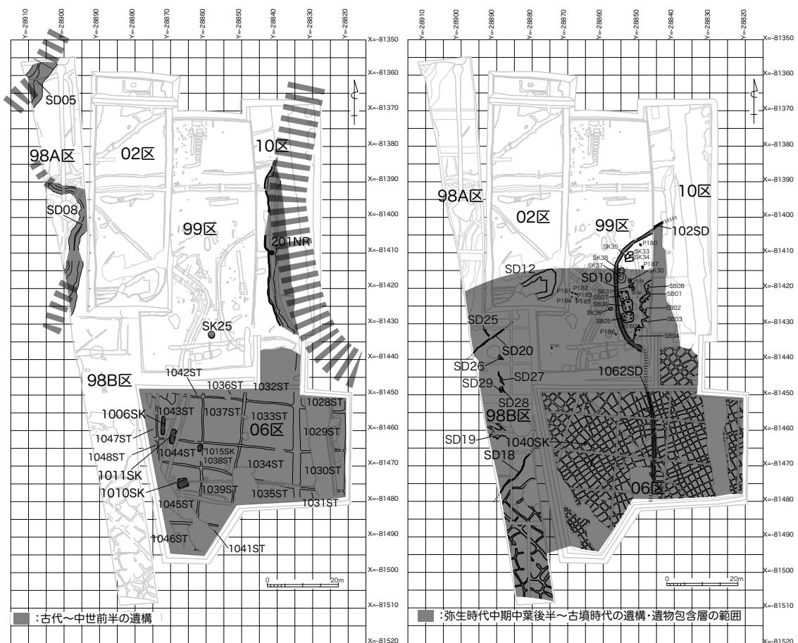
伝法寺野田遺跡の遺構変遷 (1:1,500)
