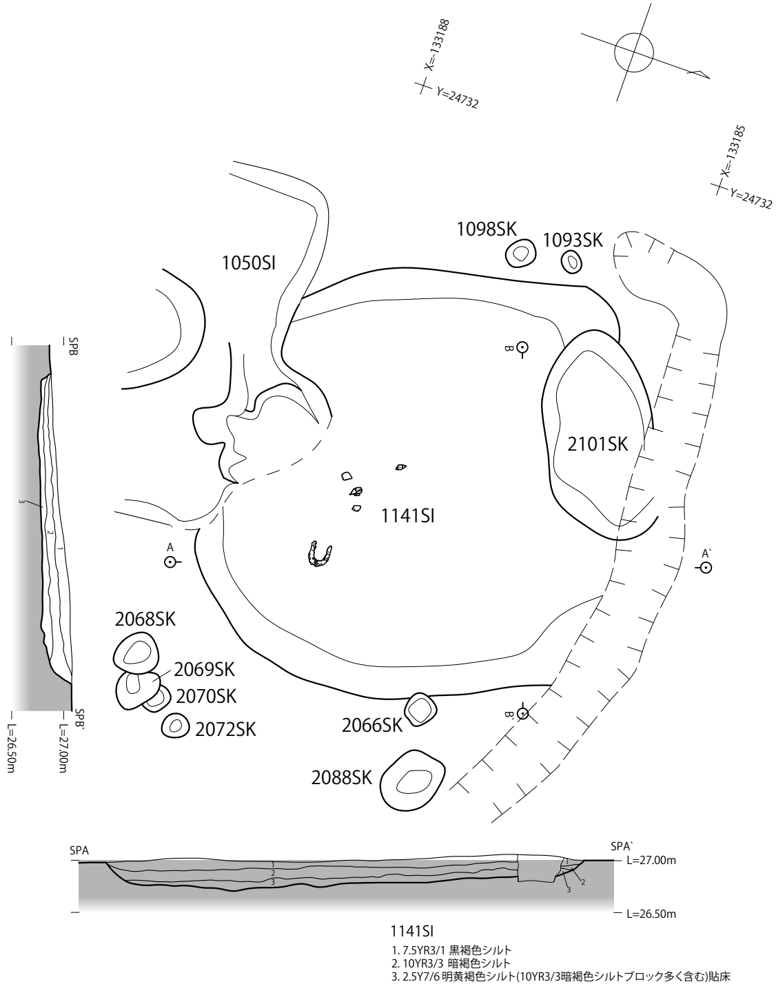
1141SI 平面・断面図 (1:50)
